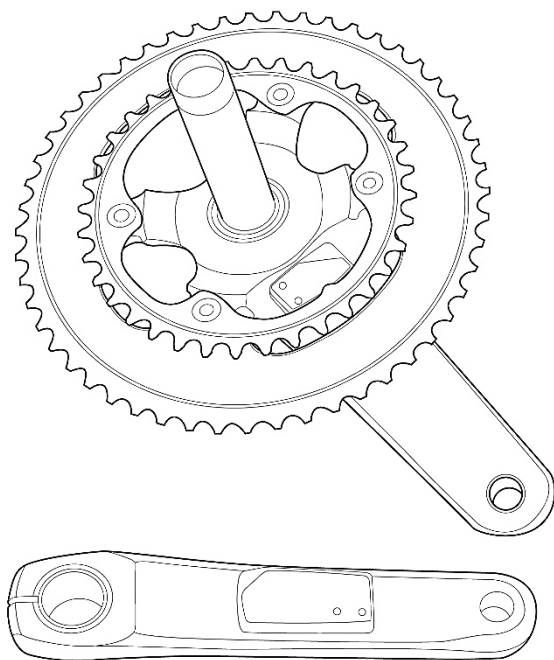
Biela derecha
