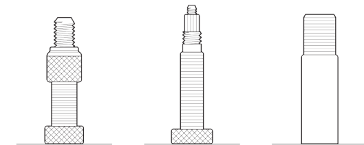
Válvula Woods / Dunlop Válvula Presta Válvula Schraeder
