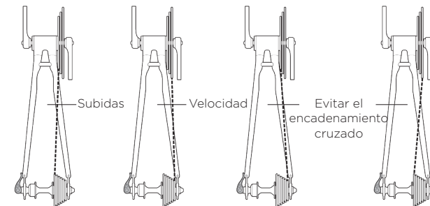
Figura 13 Engranajes traseros más grandes y delanteros más pequeños
