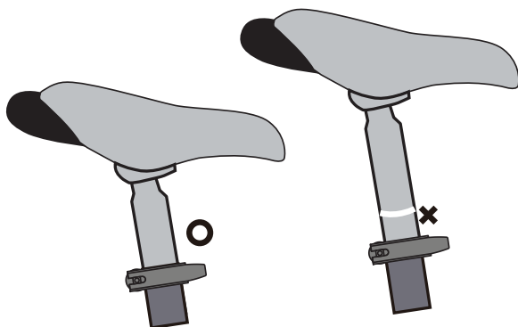
AFBEELDING 3 Plaats in het frame en zorg dat de indicatielijn voor minimale insteekdiepte op de zadelpen in het frame zit
