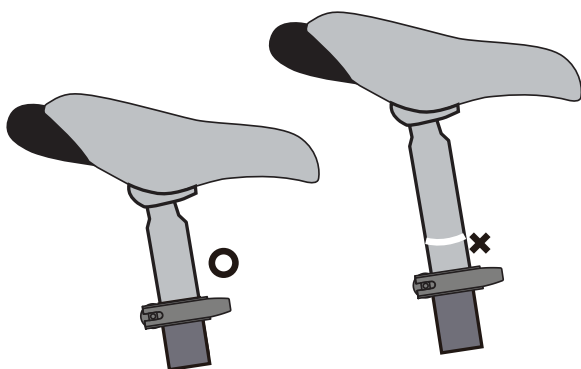
FIGURA 3 Inserimento nel telaio La linea di inserimento minima deve essere all'interno del telaio
