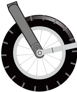
AFBEELDING 3 Vastzetten met 5-6 Nm
