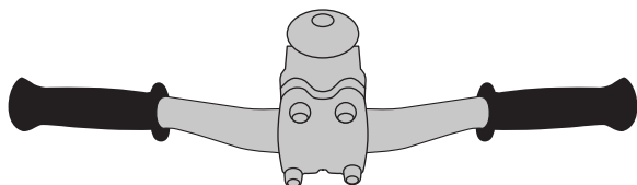
圖片 3 鎖上螺絲至5.2Nm
