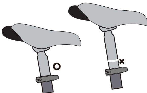
RYSUNEK 3 Punkt włożenia rury do ramy musi się znajdować w powyżej linii oznaczającej minimalną wysokość montażu
