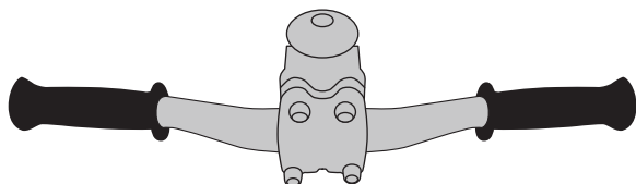
图 3 锁上螺丝至5.2Nm
