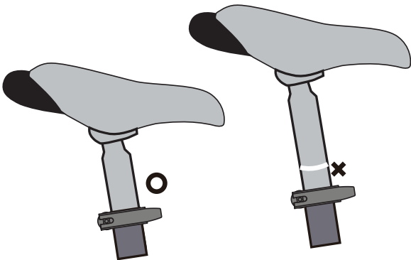
FIGURA 3 La inserción en la línea de inserción mínima del cuadro debe estar dentro de este
