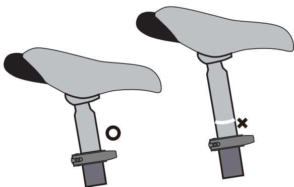
圖片 3 安裝於車架上。最 低插入長度標記需 低於車架座管上端
